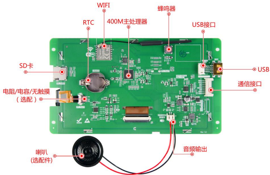
图 1-4 硬件配置图
